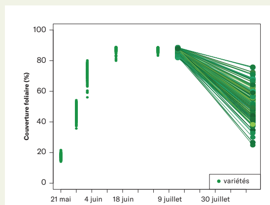
Evolution des taux de couverture mesuré par drone dans un essai de comparaison de variétés (Charmont 2018). Chaque point correspond à une variété. (figure 4)
