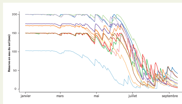
Bilans hydriques évalués par Irribet sur les différents sites d'expérimentation des variétés rhizomanie. (figure 3)
